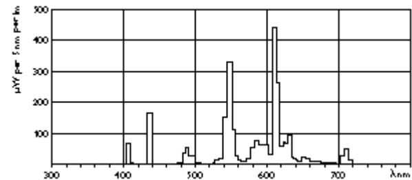
Lichtfarbe /827 MASTER PL-L/827
