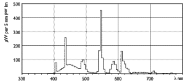
Lichtfarbe /865 MASTER PL-L/865
