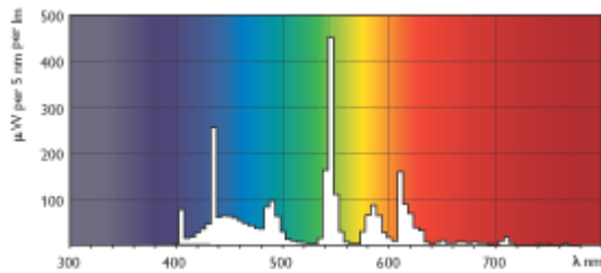
Lichtfarbe /865 MASTER PL-L/865
