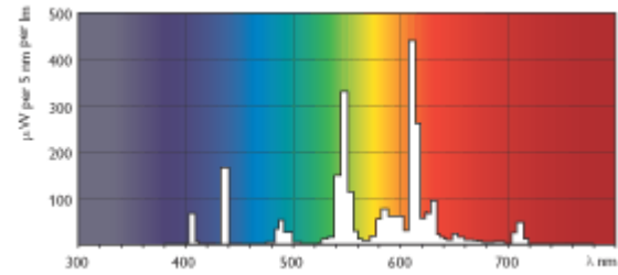
Lichtfarbe /827 MASTER PL-L/827
