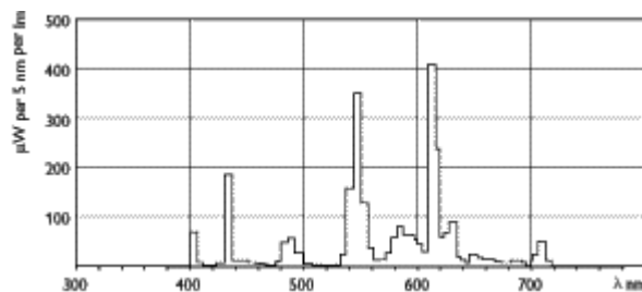
Lichtfarbe /830 MASTER PL-L/830
