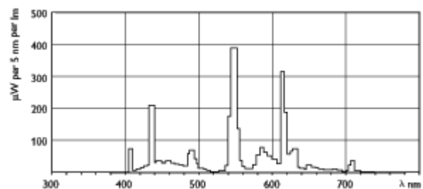
Lichtfarbe /840 MASTER PL-L/840
